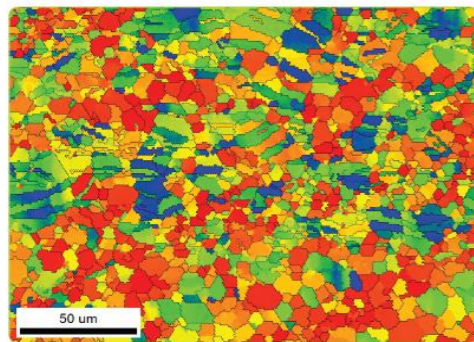
EBSD mapping
